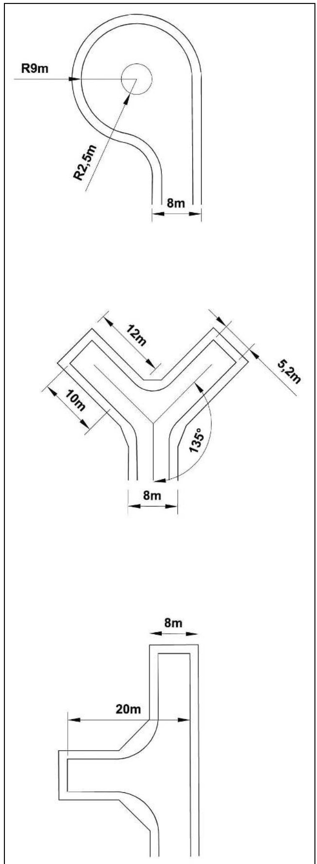
Caractéristiques dimensionnelles minimales des dispositifs d'aires de retournement
